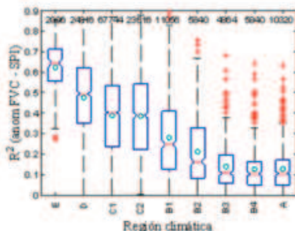
Figura 11. Distribución de los valores de R^2 (correspondientes a la figura 10) para las regiones climáticas de España.
