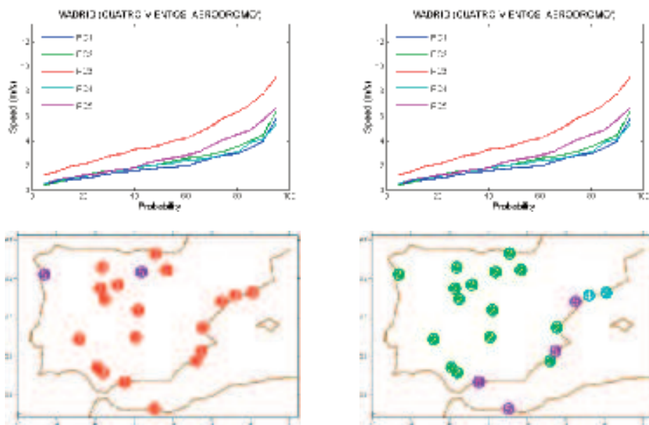
Figura 4. Frecuencias acumuladas de velocidad del viento asociadas a valores (a) positivos y (b) negativos de las componentes principales de Z1000 para Madrid. Componentes principales dominantes obtenidos para los valores más altos de frecuencias acumuladas de velocidad del viento: (c) valores positivos y (d) valores negativos.
