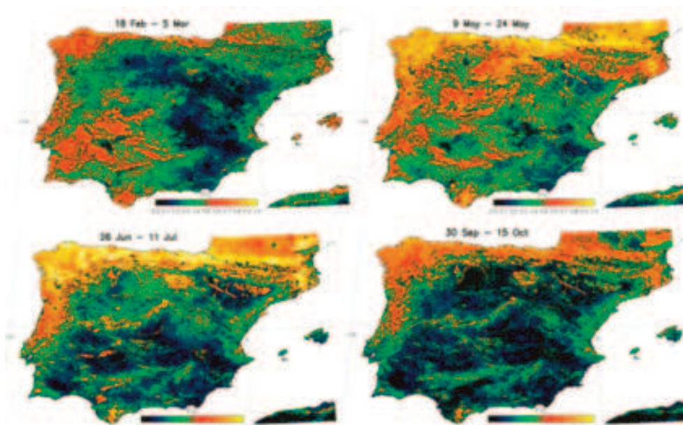
Figura 1. Valores medios de la cobertura vegetal (FVC) a lo largo de 11 años correspondientes a cuatro periodos diferentes del año.
