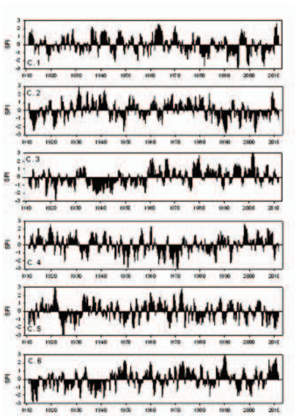
Figura 2. Evolución de las series de SPI correspondientes a los seis componentes extraídos.
