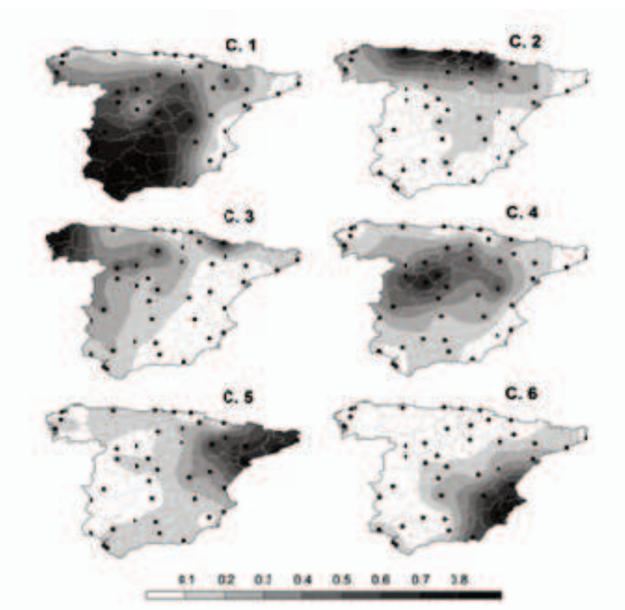
Figura 3. Distribución espacial de las cargas factoriales correspondientes a los seis componentes principales extraídos.
