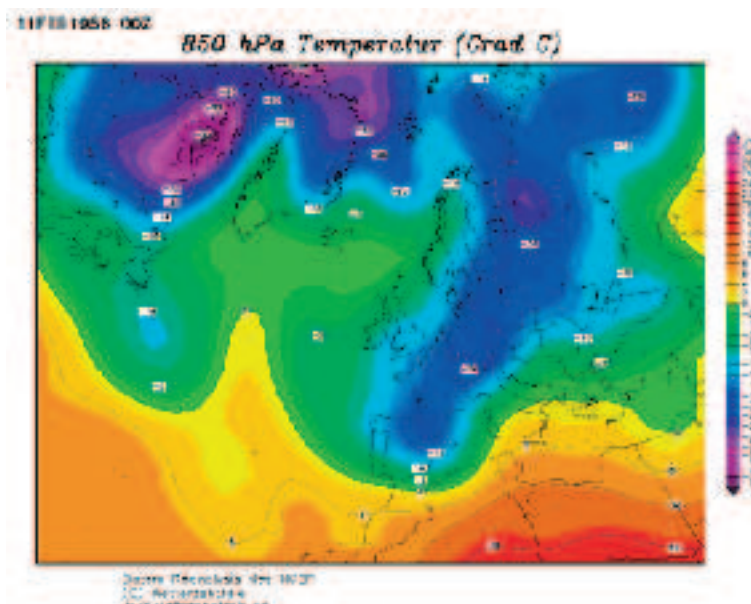
Figura 4. Temperatura (° C) en el nivel de 850 hPa del día 11 de febrero de 1956. (Reanálisis NCEP/NCAR).
