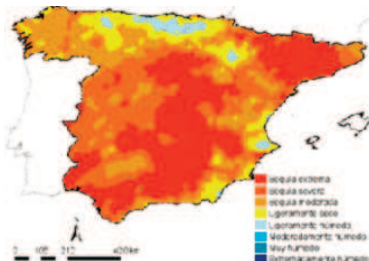
Figura 3. Distribución espacial de la sequía en la España peninsular correspondiente al periodo enero-diciembre de 2005, a partir del SPI-12: Extremadamente húmedo ( >2.0 ), Muy húmedo ( 1.5 a 1.99 ), Moderadamente húmedo ( 1.0 a 1.49 ), Ligeramente húmedo ( -0.99 a 0.0 ), Ligeramente seco ( 0 a 0.99 ), Sequía moderada ( -1.49 a 1.0 ), Sequía severa ( -1.99 to 1.5 ), y Sequía extrema ( <-2.0 ).
