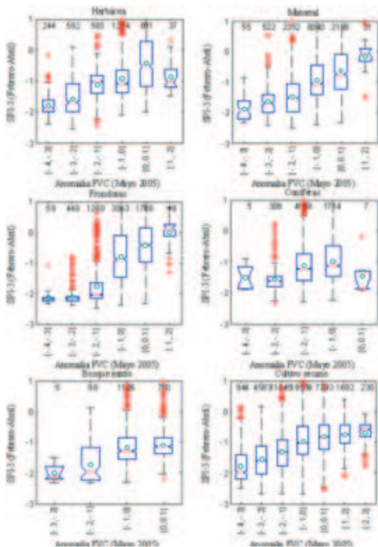
Figura 7. Distribución de los valores de SPI-3 (febrero-abril) en función de la anomalía en la cobertura vegetal (FVC) del mes de mayo, para varios tipos de cubierta diferente. Las cajas identifican los percentiles 25, 50 y 75, los círculos el valor medio y el símbolo (+) valores anómalos. La cifra en la parte superior indica el número de píxeles en cada clase.
