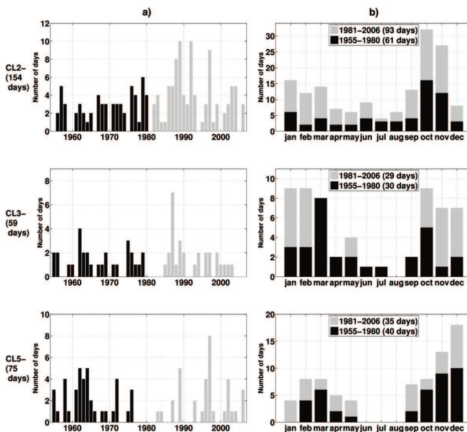
Figura 6. Como la figura 5, pero para las clases correspondientes a las fases negativas de los modos encontrados.
